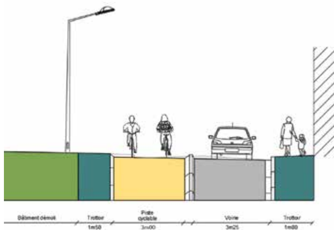
Projet de redéfinition du partage de la voirie avec piste bidirectionnelle au niveau du quai aux Arbres.
